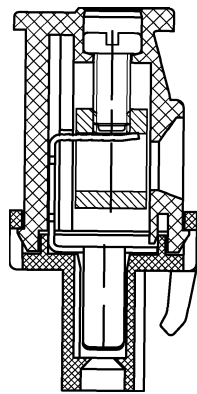
SECTION:A-A
