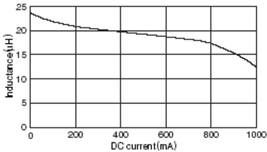
SDS5014M-220M-LF
