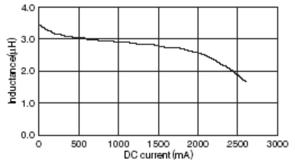
SDS5014M-2R7M-LF
